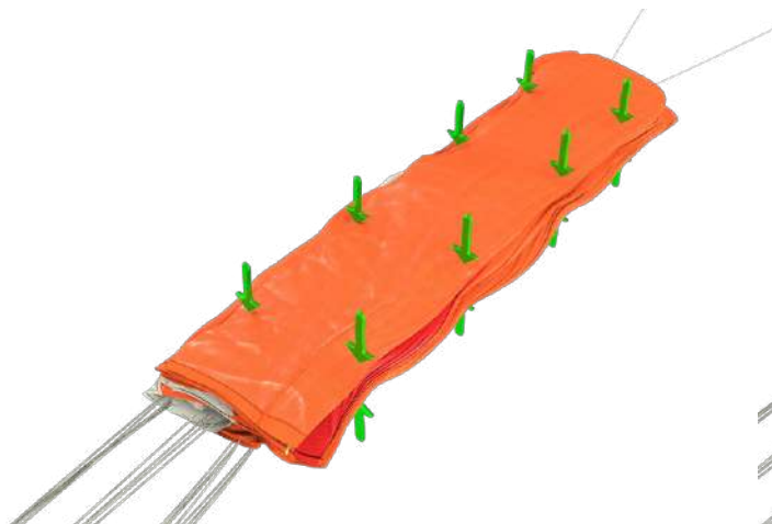
Figure 21 – Mesure la profondeur du P.O.D., en partant de la base de la voileure.
